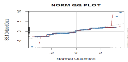
Fig 6 USD/NGN Q-Q plot:
